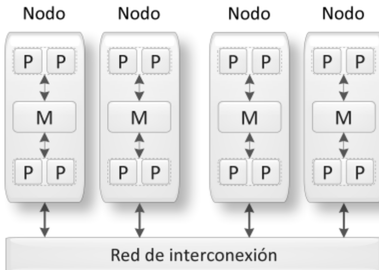
Figura 2.3: Plataforma de memoria híbrida.
